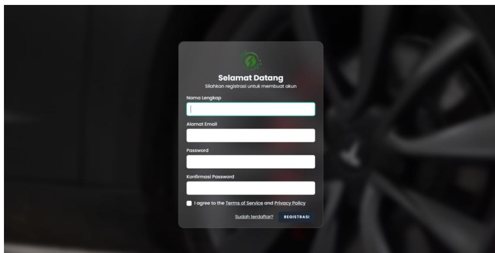
Gambar 14. Implementasi Register
